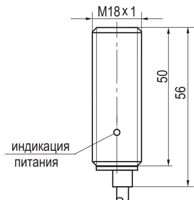
Габаритный чертеж
